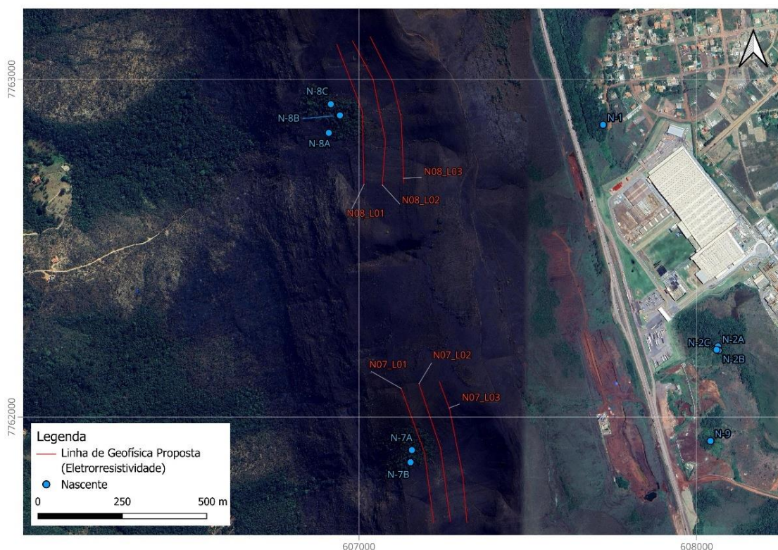
Figura 4: Linhas propostas para estudo geofísico pelo método de eletrorresistividade.
